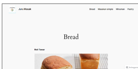
Gambar 4. Hasil Pelatihan.
